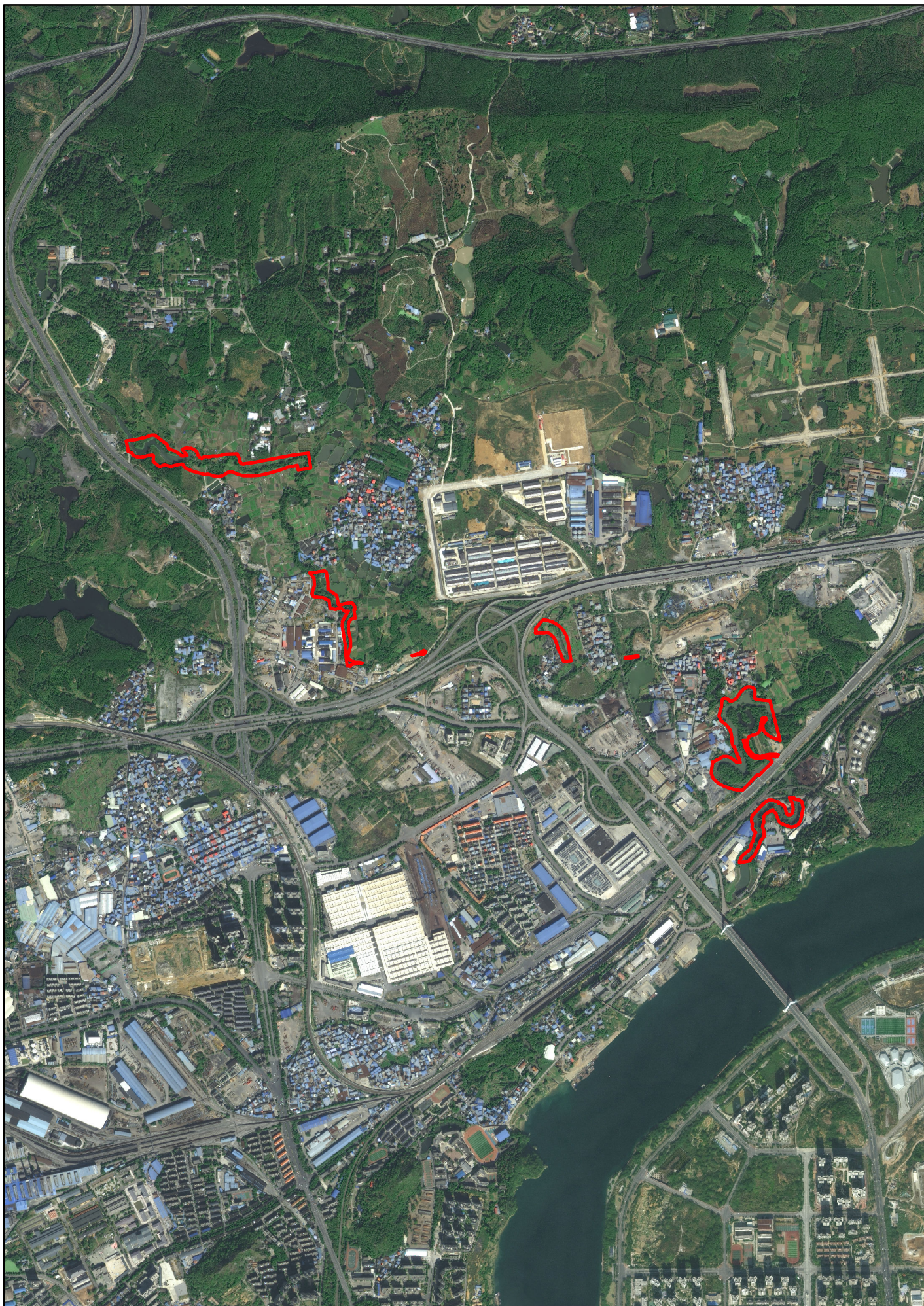
香兰河流域生态综合治理工程项目（柳北区A地块）影像示意图
