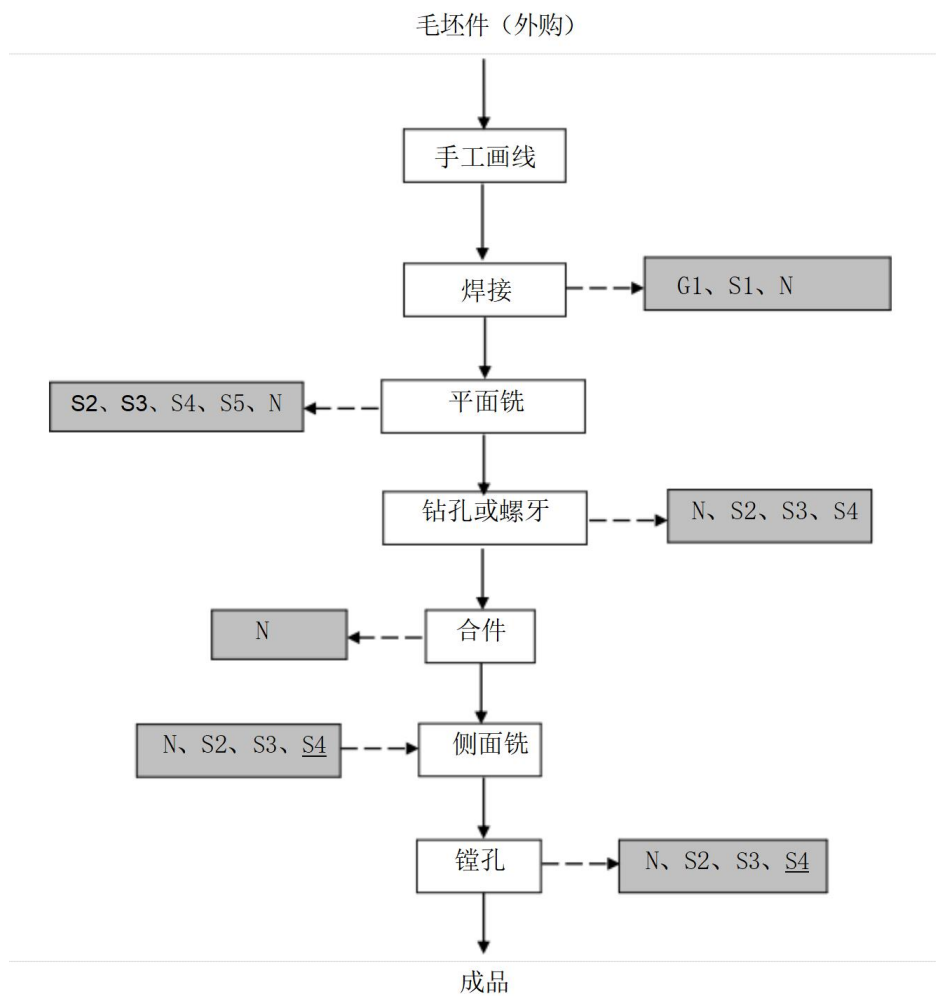
图2 前后摆动支架生产工艺流程及产污环节图
