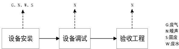
施工工艺流程及产污环节图
