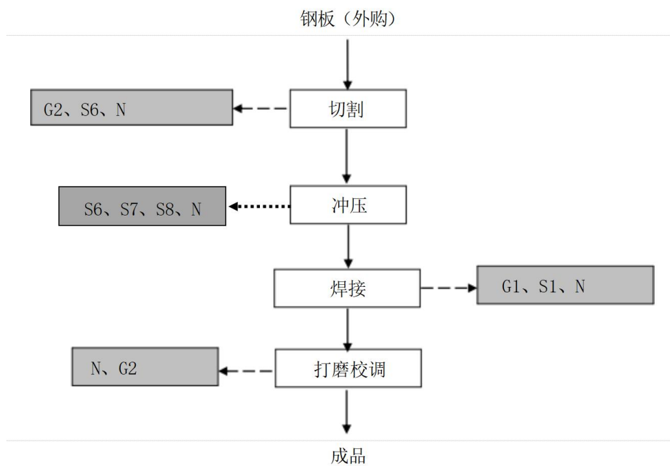
图 3 非标成套设备、汽车零部件生产工艺流程及产污环节图
