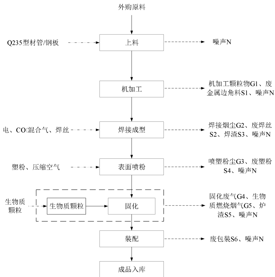
项目生产工艺及产污流程图
