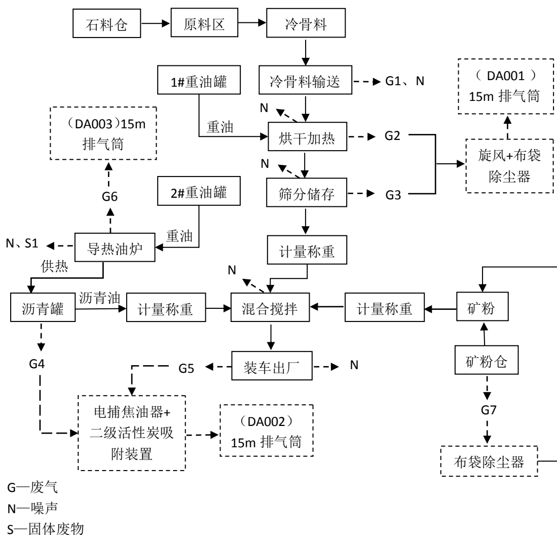
项目生产工艺流程及产污环节图
