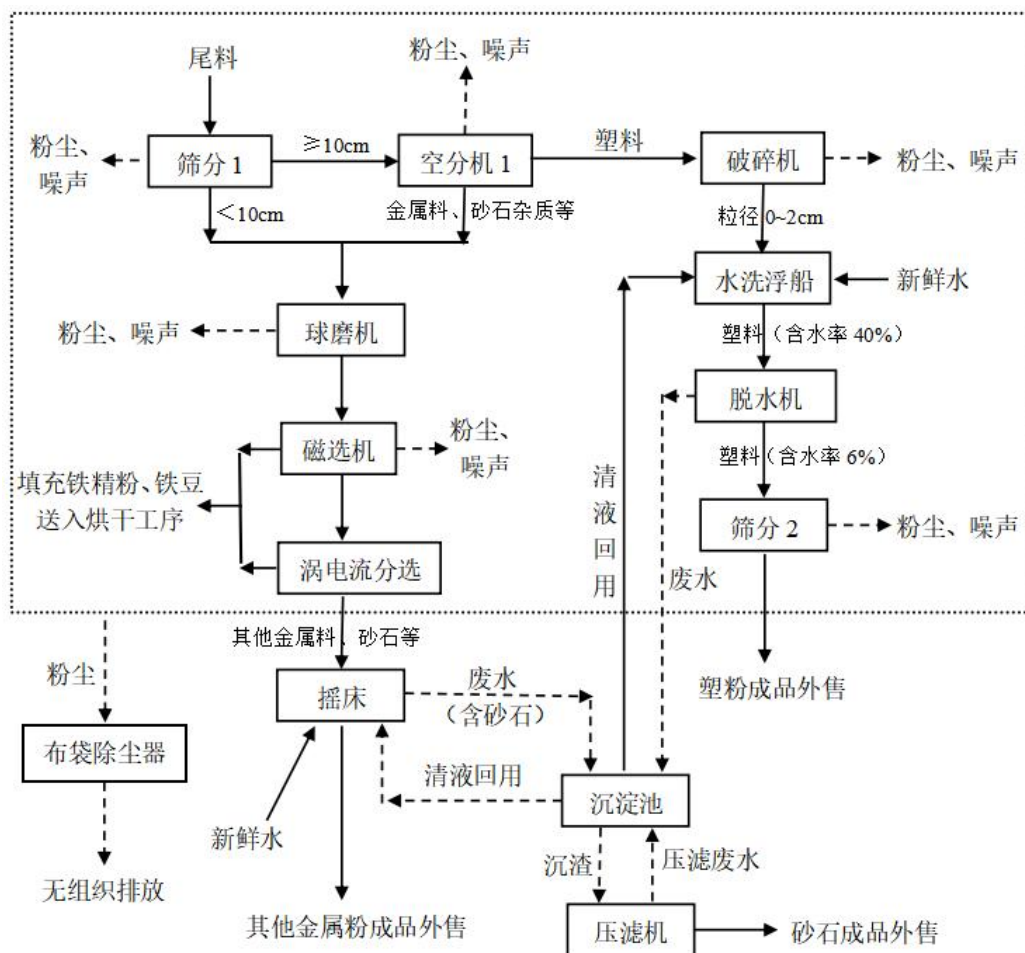
项目尾料加工线生产工艺流程及产污节点图
