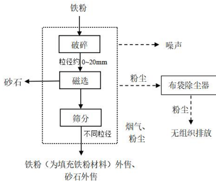
项目铁粉加工线生产工艺流程机产污节点图
