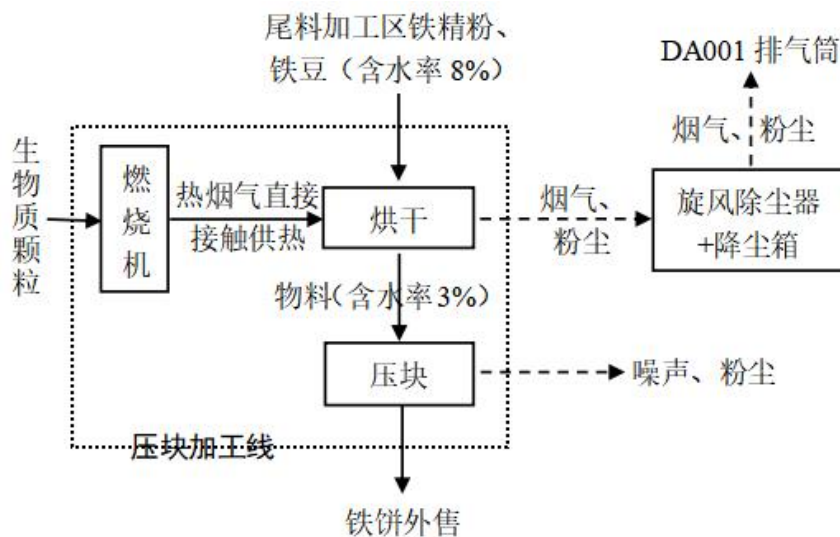
项目压块加工线生产工艺流程机产污节点图
