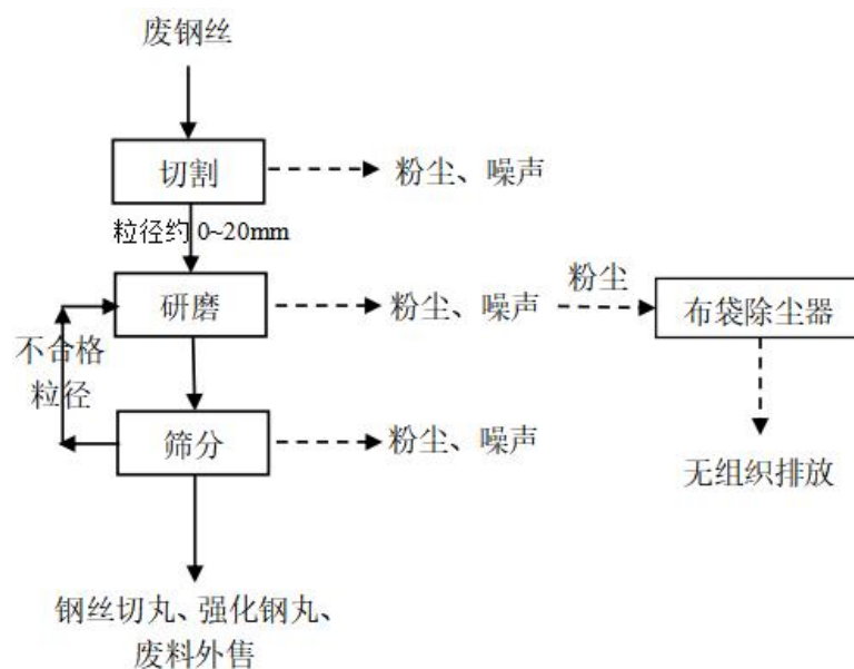
项目金属磨料加工线生产工艺流程机产污节点图
