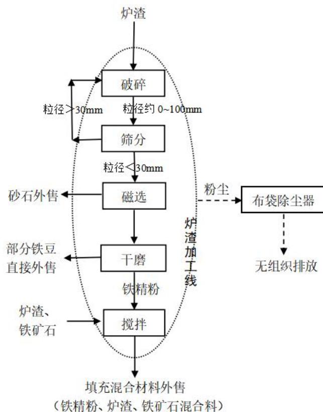
项目炉渣加工线生产工艺流程及产污节点图
