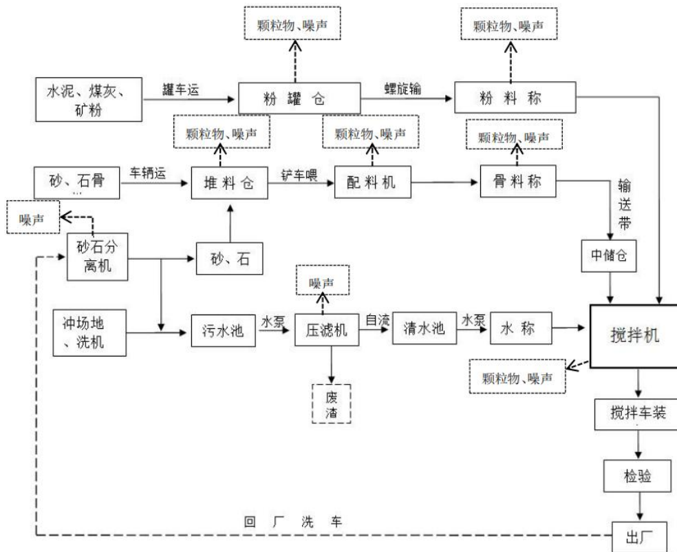
项目混凝土生产工艺流程及产污节点图
