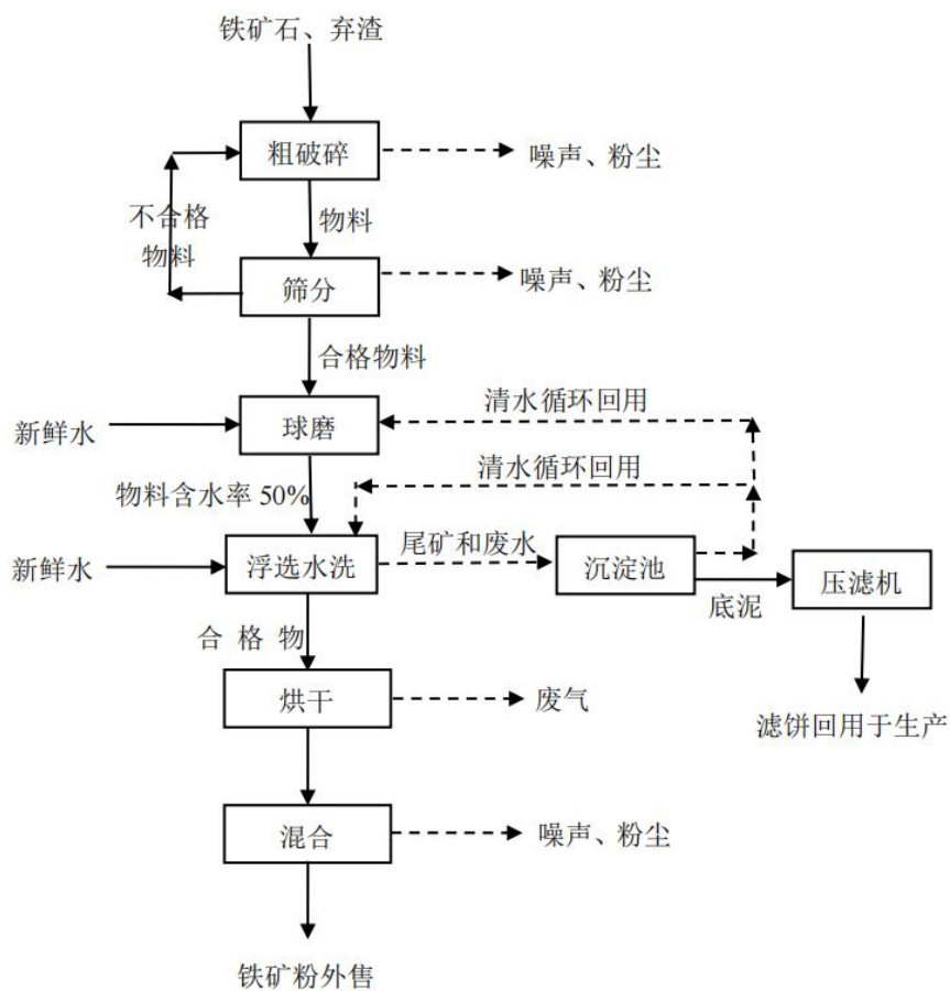
项目铁矿粉生产工艺流程及产污节点图
