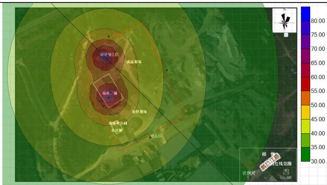
图4-2 项目噪声预测等声线图单位:dB(A)
